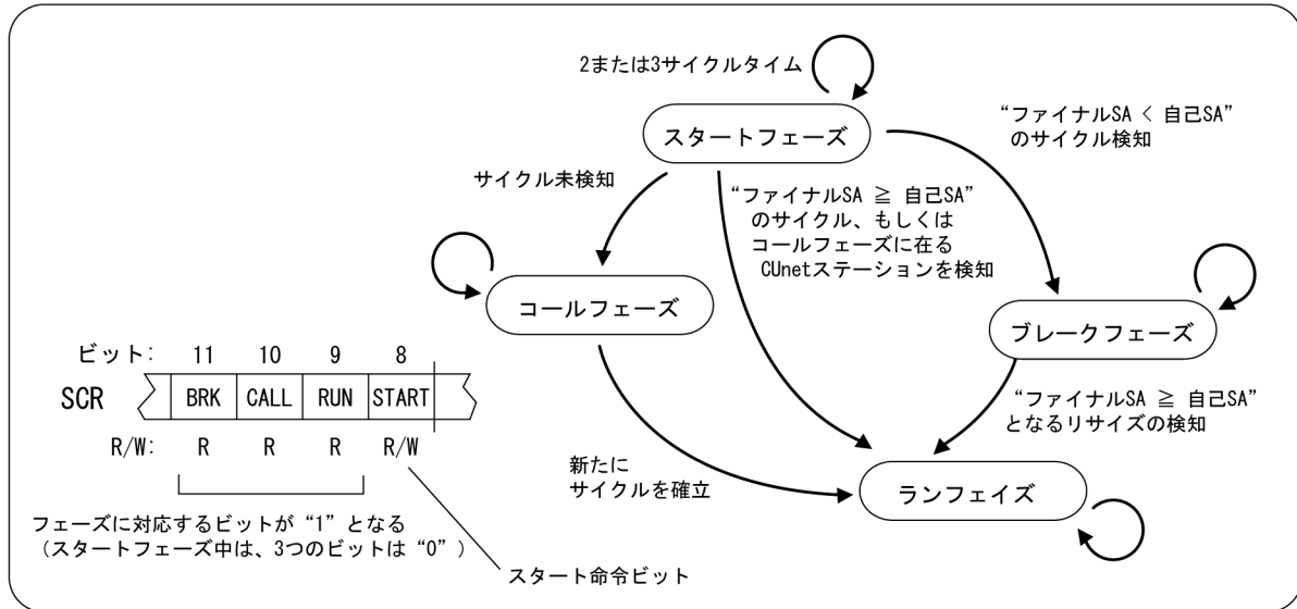
図4.2 MKY43のフェーズ遷移とSCRの対応ビット
