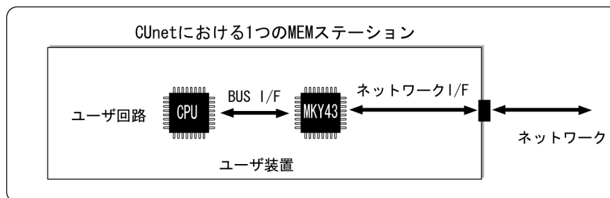
図1.1 MKY43を搭載したCUnetステーション (MEMステーション)
