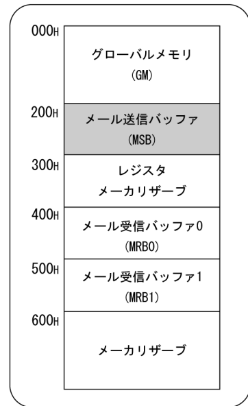
図4.22 メール送信バッファ
