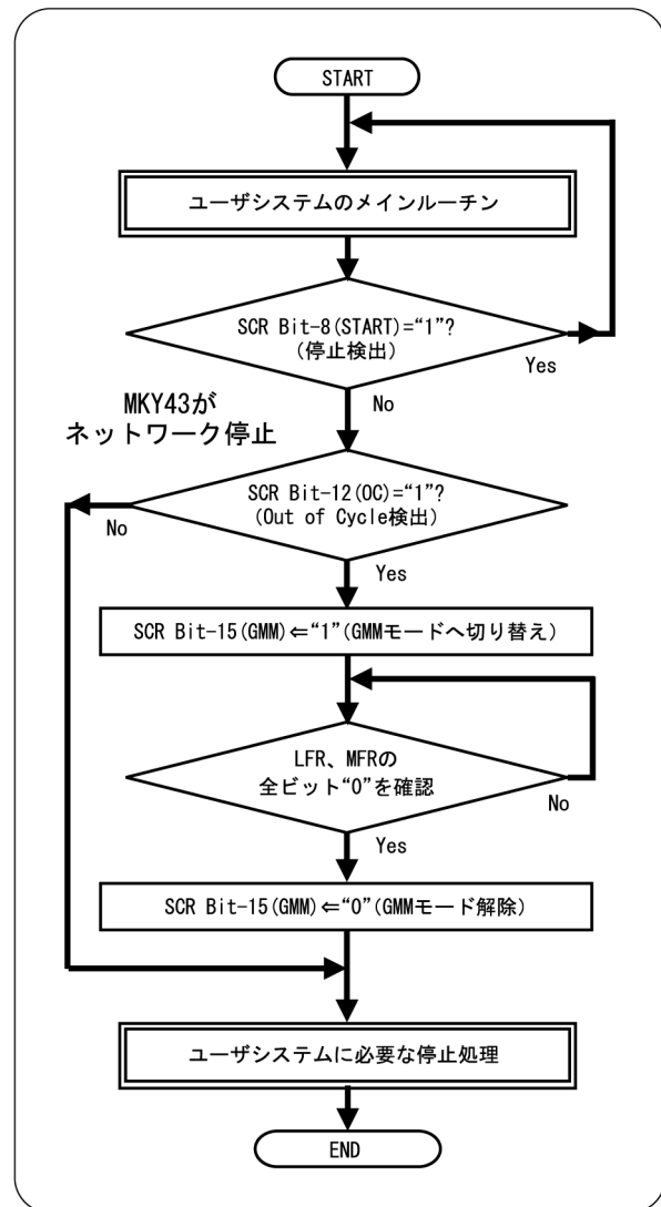
付図1 ポーリングによる停止時の処理例
