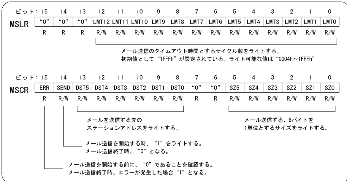
図4.23 MSLRとMSCRの操作
