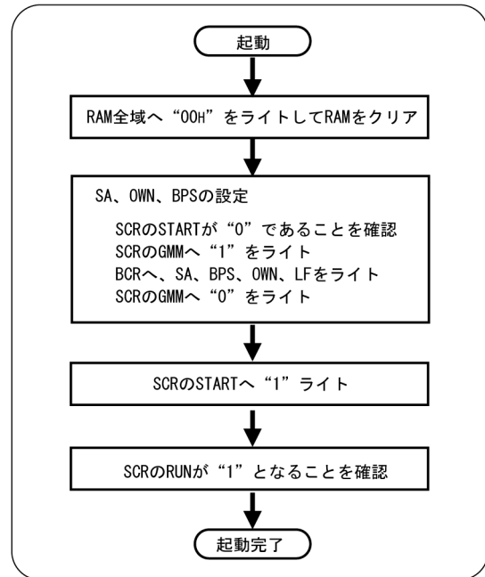
図4.1 起動のアルゴリズム
