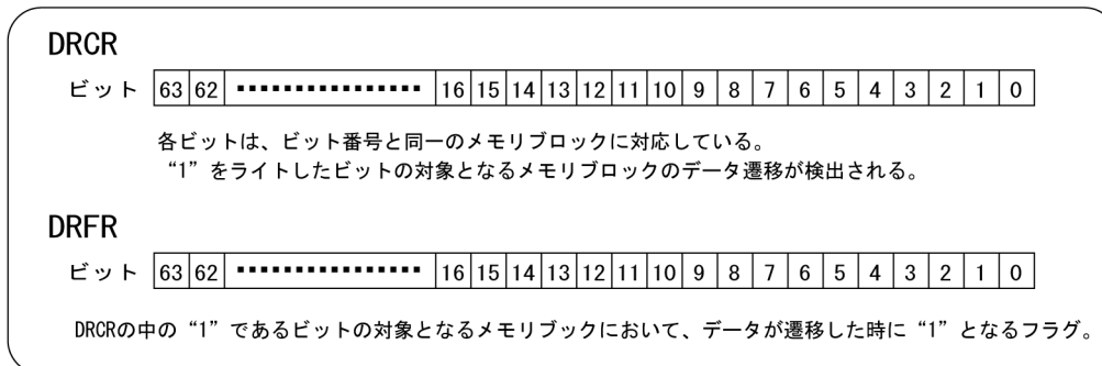
図4.16 64ビットのDRCRとDRFR
