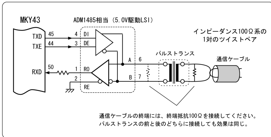
図3.3 推奨のネットワーク接続
