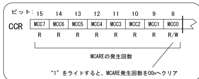
図4.32 CCRのMCARE発生回数
