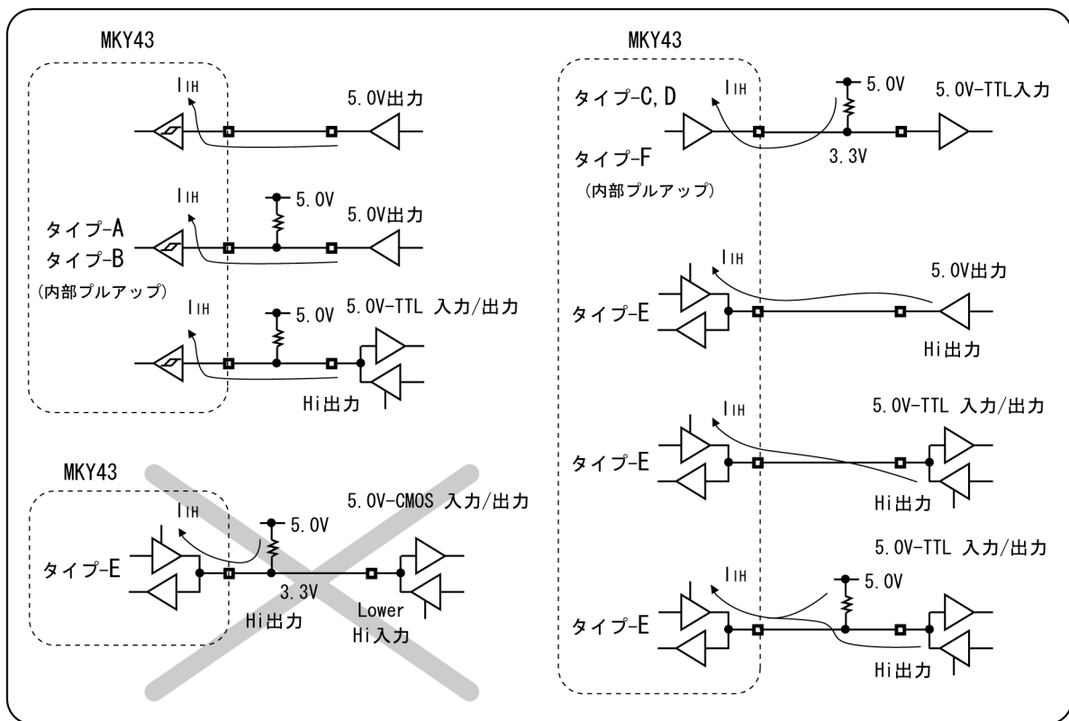
図3.1 リークの生じる接続
