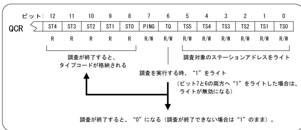
図4.35 各MEMステーションのモード調査
