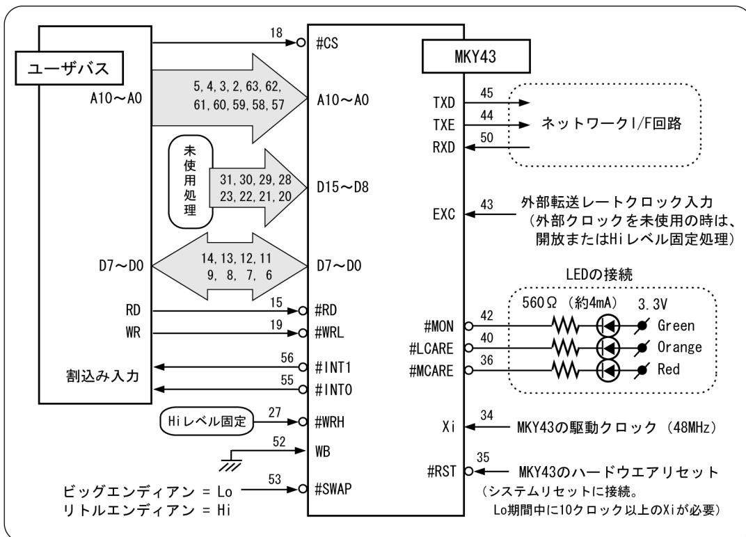
図3.8 8ビットユーザバスとの接続
