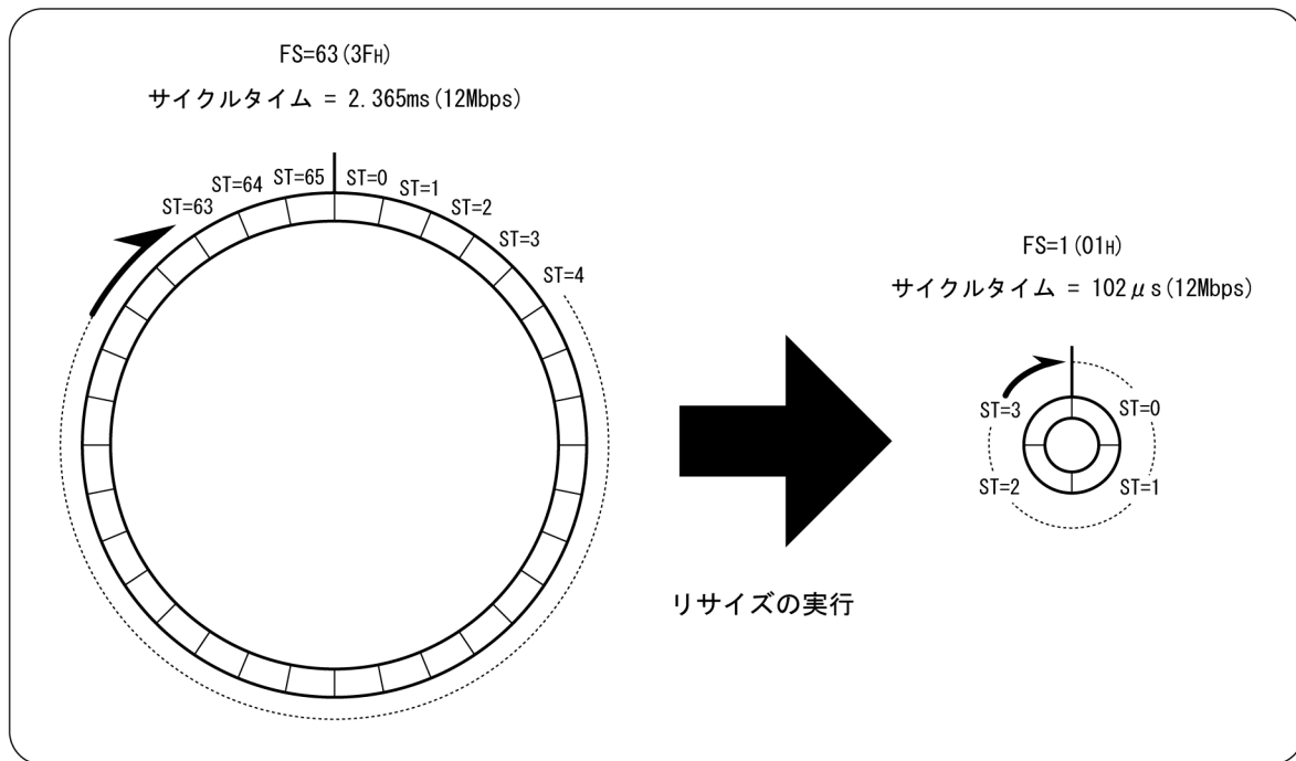
図4.26 リサイズ
