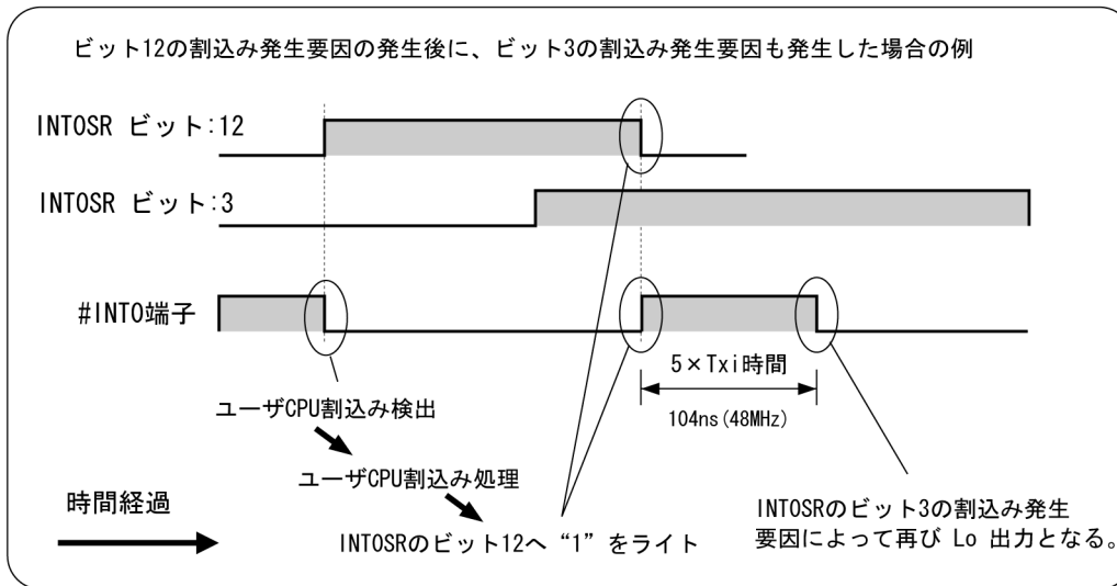
図4.40 リトリガ機能の動作例
