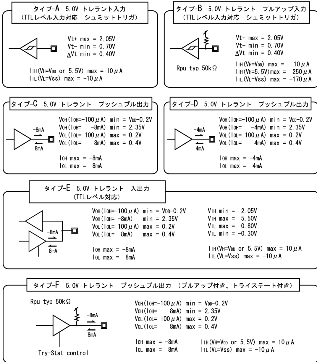
図2.2 MKY43の入出力回路形式における端子電気的特性
