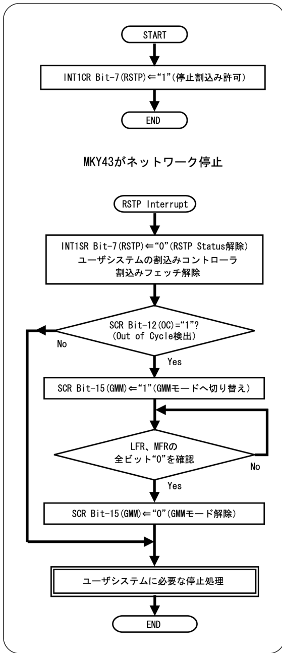
付図 2 割り込みを利用した停止時の処理例(1)
