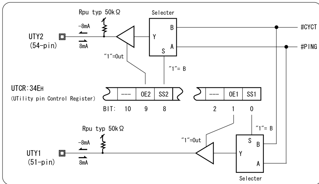
図3.5 UTY1端子、UTY2端子の制御
