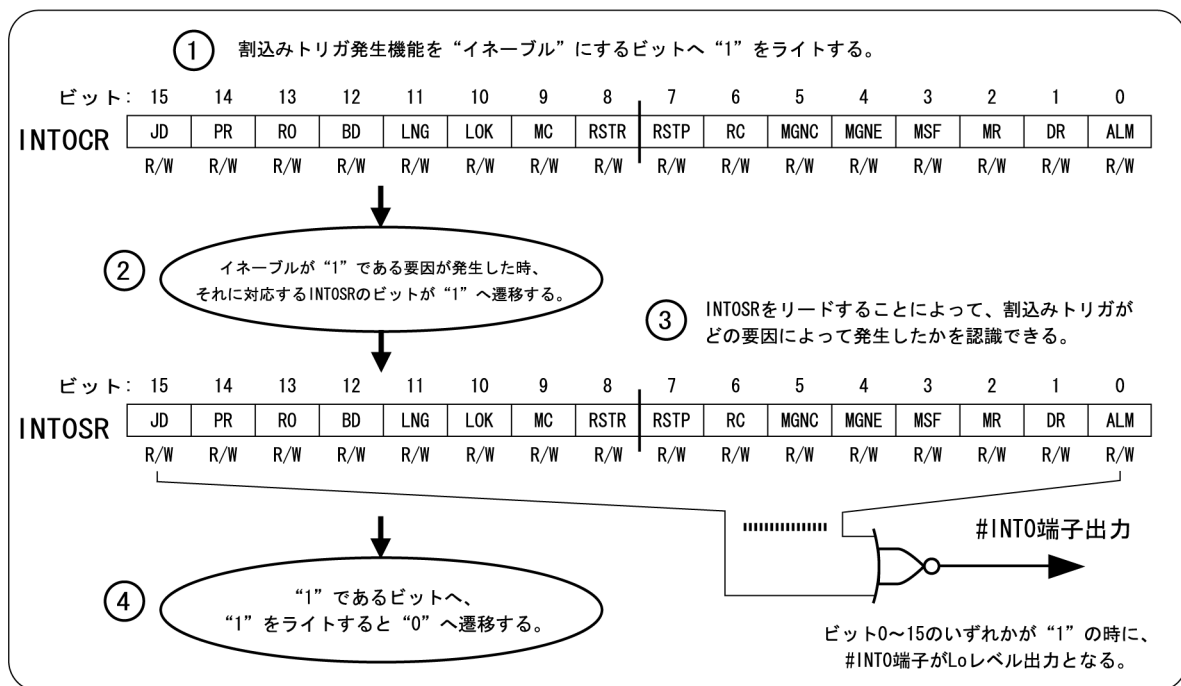
図4.38 割込みトリガ発生機能
