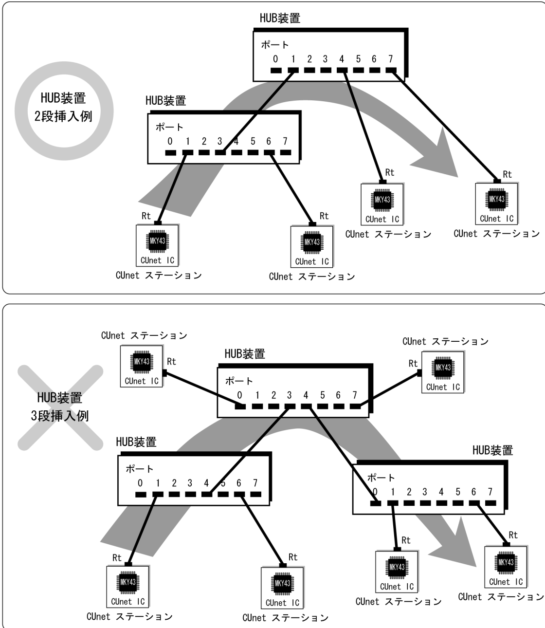
図4.36 HUB挿入可能段数
