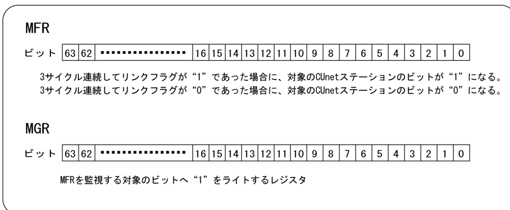
図4.14 64ビットのMFRとMGR
