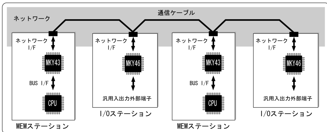
図1.4 I/Oステーションを接続したCUnet
