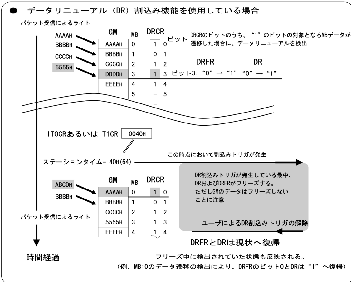
図4.17 時間経過に対するデータリニューアル検出の概要
