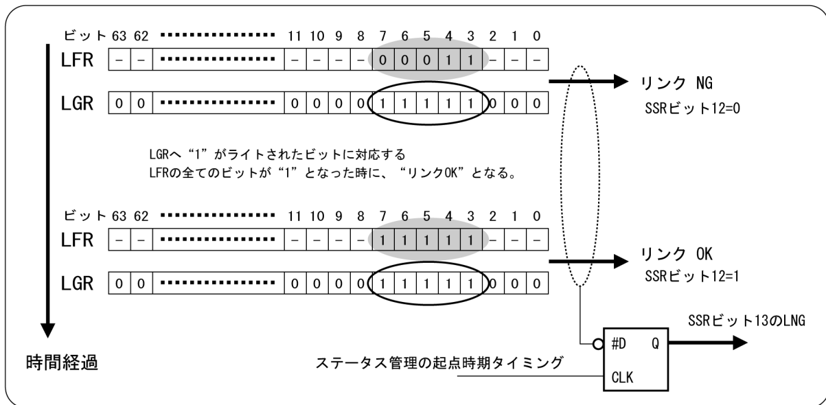
図4.13 LGRによるLFRの監視
