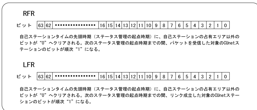
図4.11 64ビットのRFRとLFR
