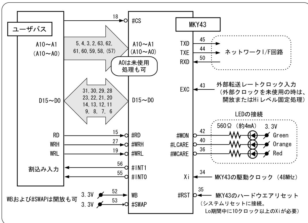
図3.7 16ビットユーザバスとの接続
