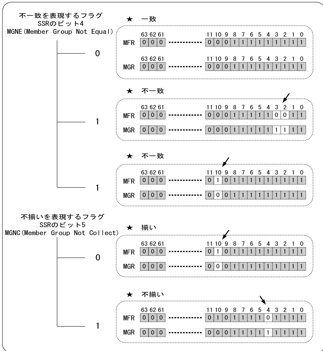
図4.15 MGRによるMFRの監視とSSRのビット状態
