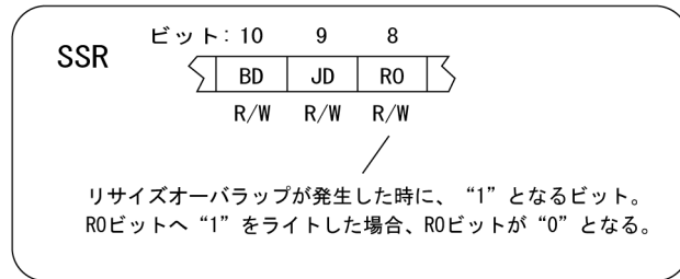
図4.28 SSRのROビット
