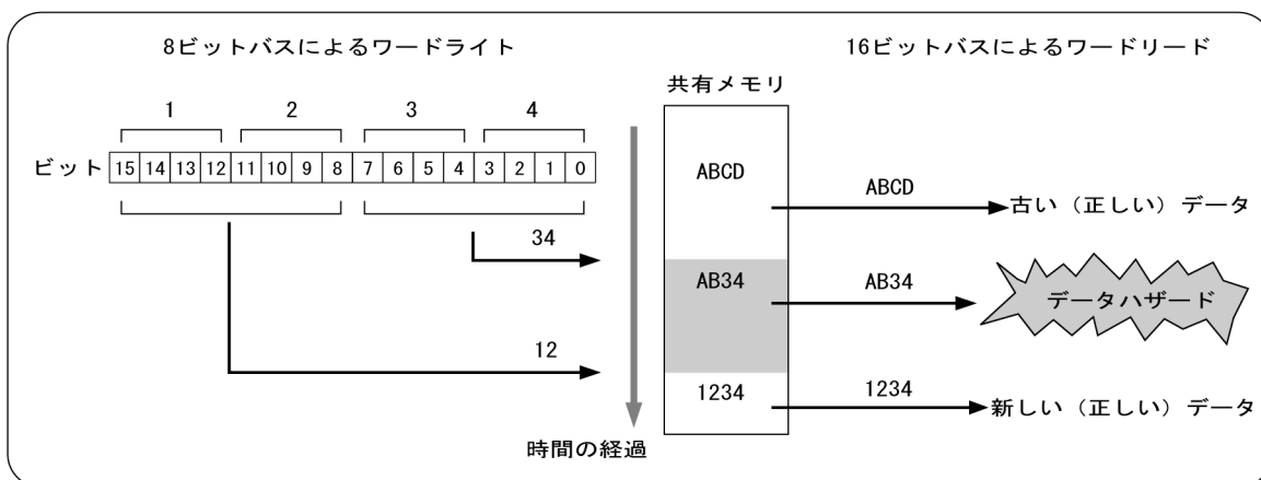
図4.8 ライトの際に発生するデータハザード
