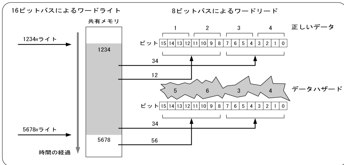
図4.7 データハザード発生メカニズム
