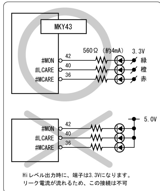
図3.4 LED表示用端子の接続例
