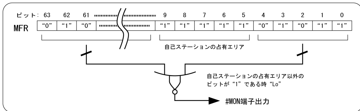
図4.33 #MON端子への出力例
