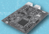
MKY43 搭載マイコンボード NFS-CUNET
