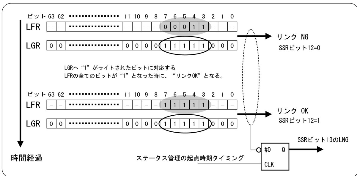
図 5.11 LGRによるLFRの監視
