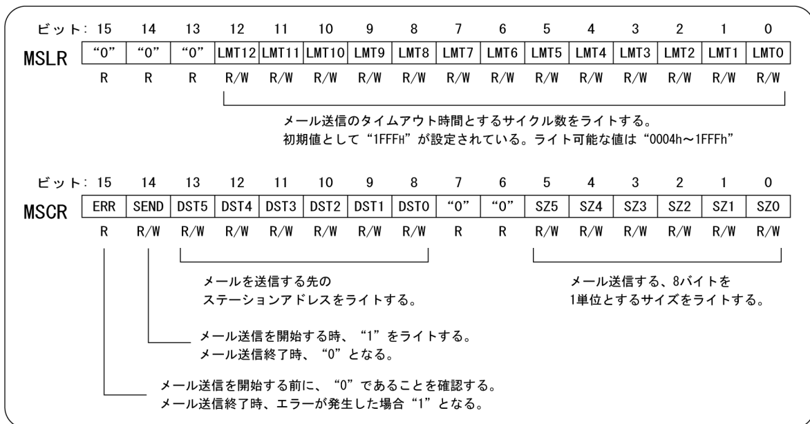
図 5.21 MSLR と MSCR の操作
