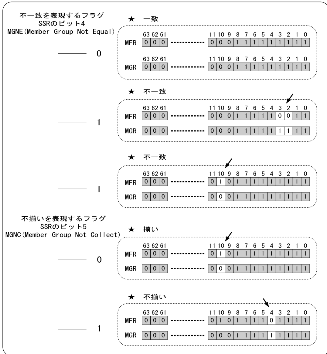
図 5.13 MGR による MFR の監視と SSR のビット状態
