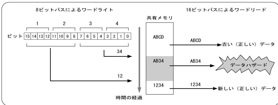
図 5.8 ライト時に発生するデータハザード
