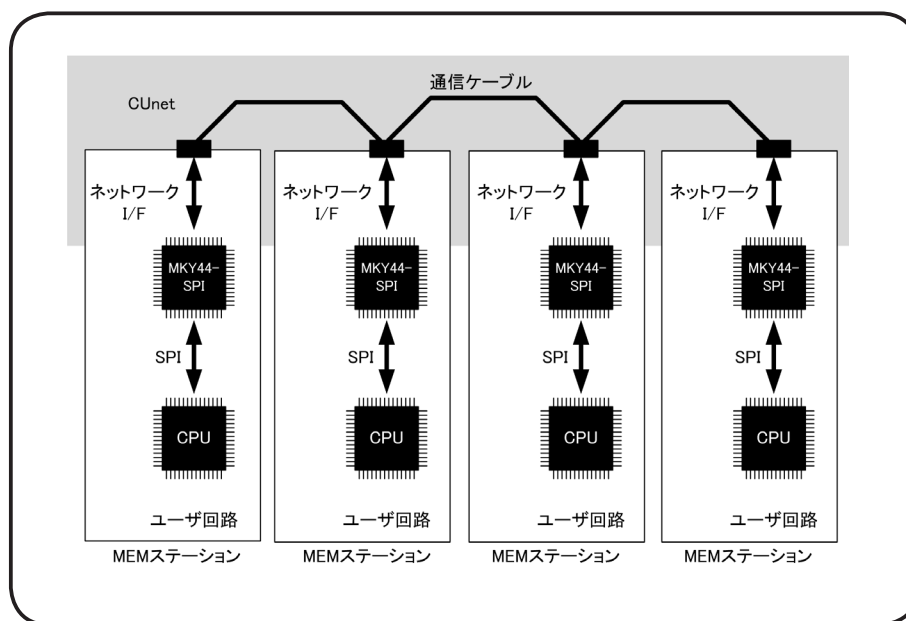
図 1.2 4 つの MEM ステーションを接続した CUnet 構成
