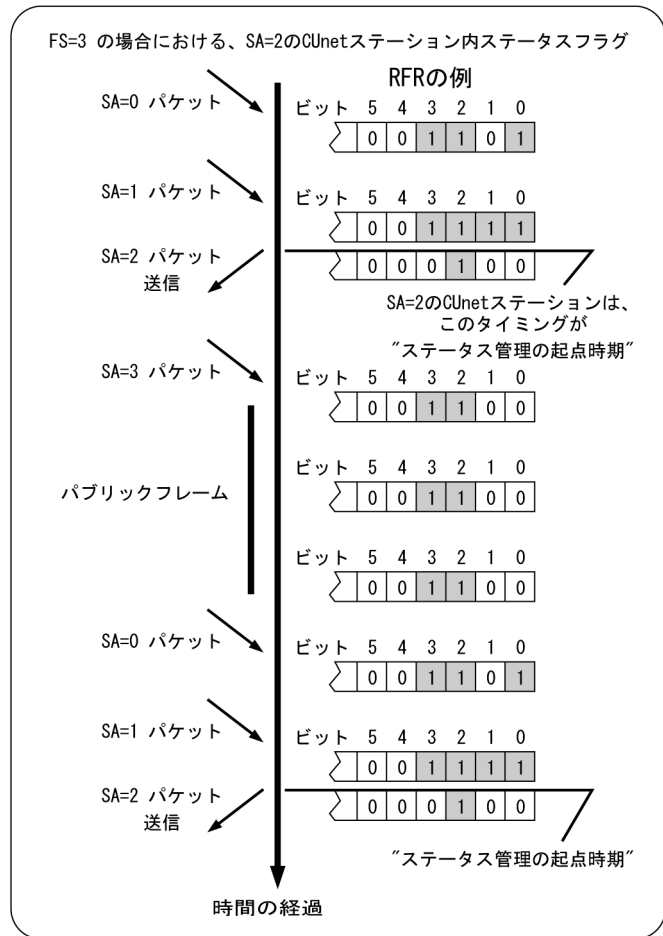
図 5.10 ステータス管理の起点時期
