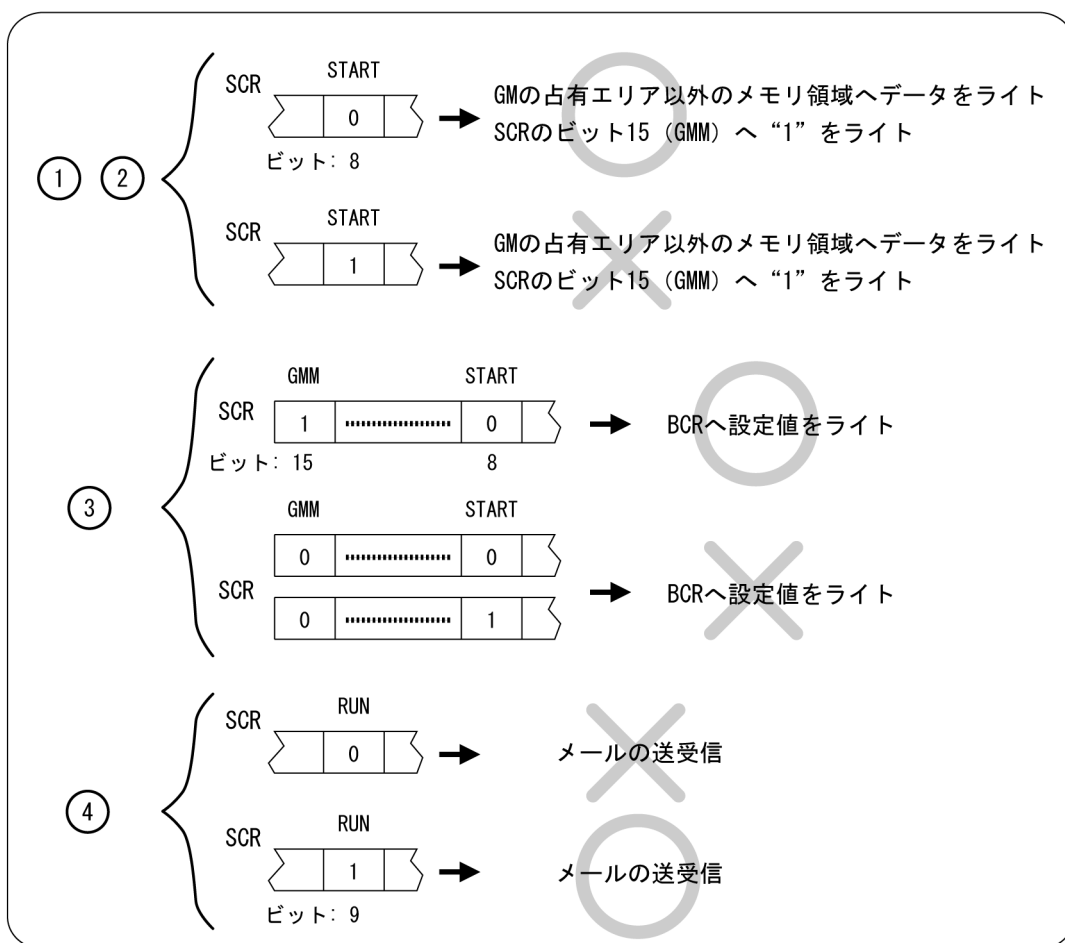
図 5.3 ライトプロテクト
