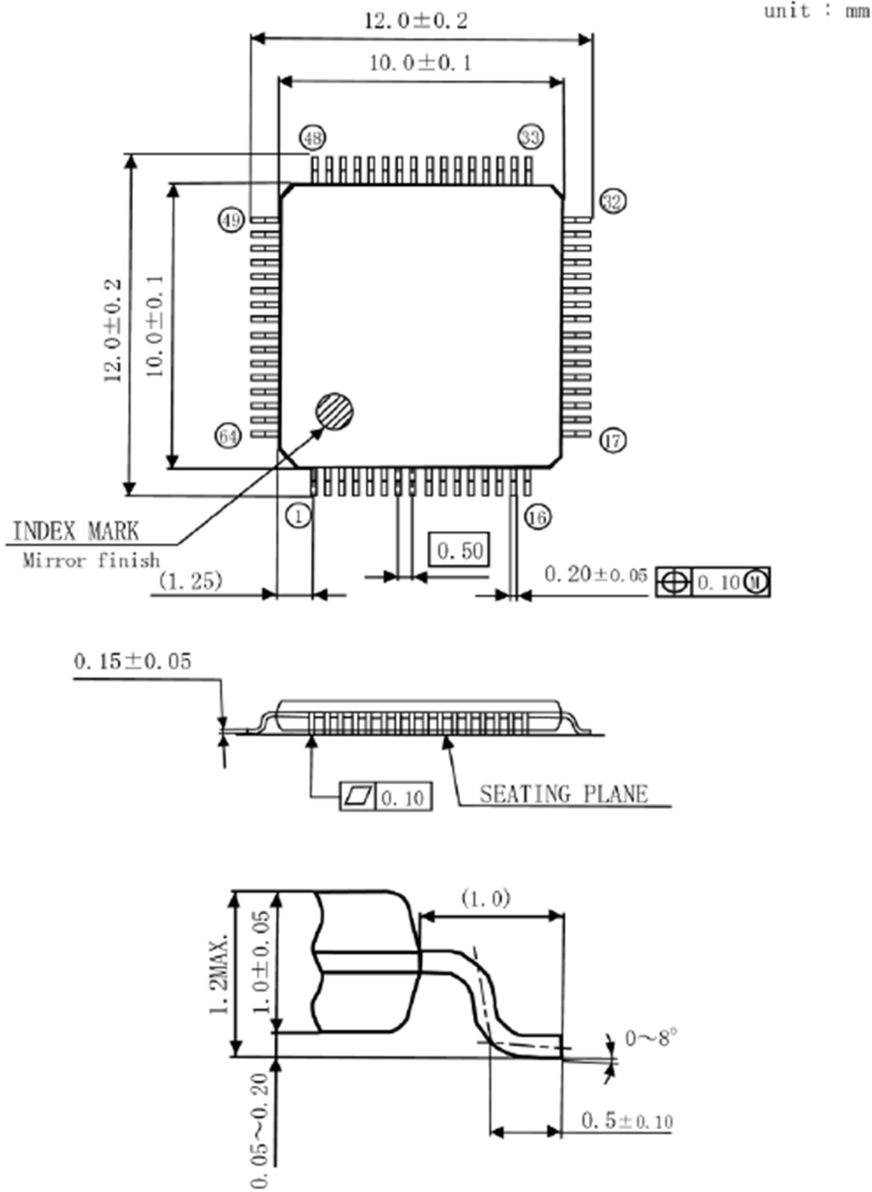
図8.1 外形寸法図
