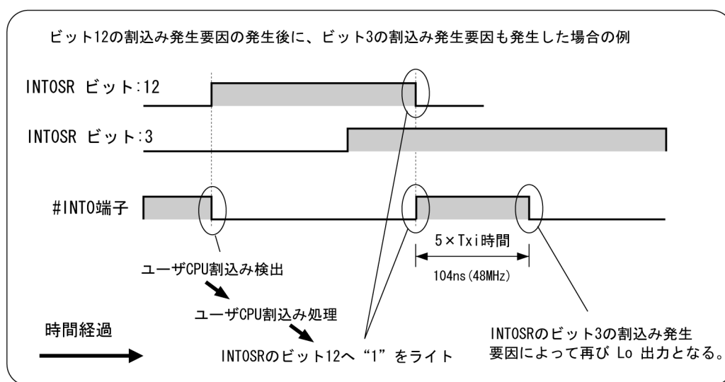
図 5.38 リトリガ機能の動作例
