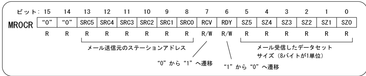
図 5.18 MRBO へデータセットを格納した時の MROCR
