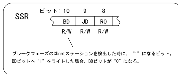
図 5.27 SSR の BD ビット
