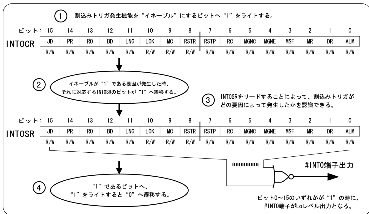
図 5.36 割込みトリガ発生機能
