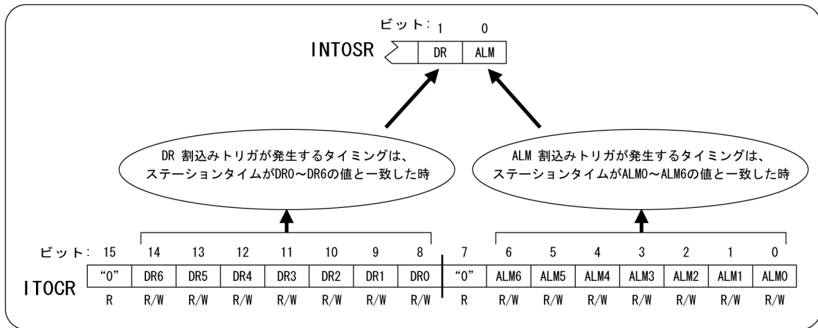
図 5.37 DR 及び ALM 割込みトリガ発生タイミング
