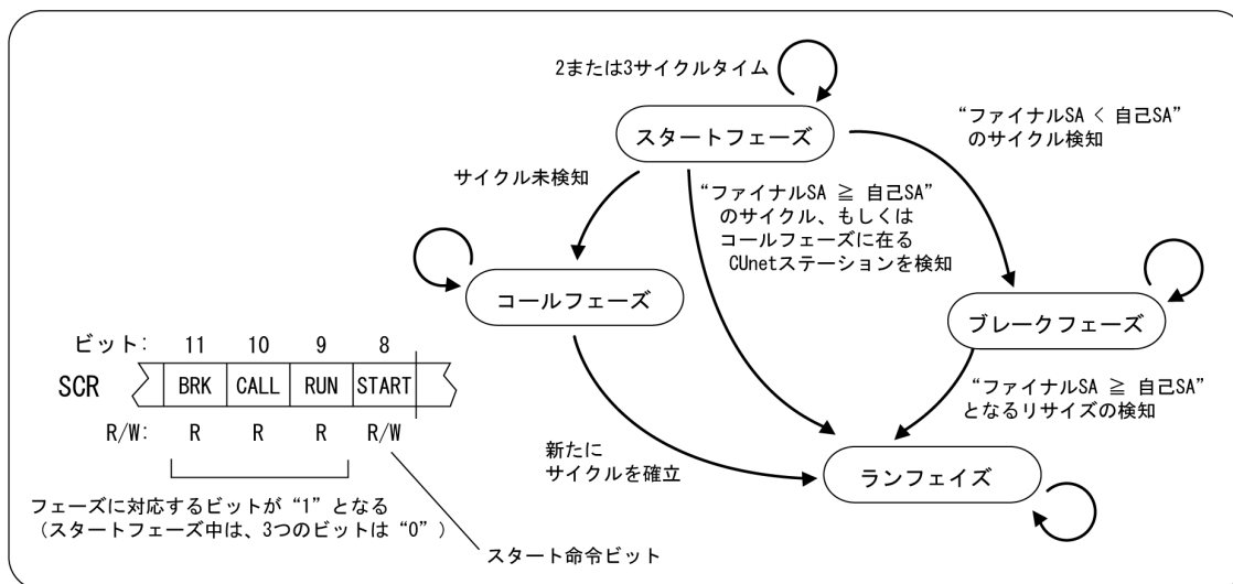
図 5.2 MKY44-SPI のフェーズ遷移と SCR の対応ビット
