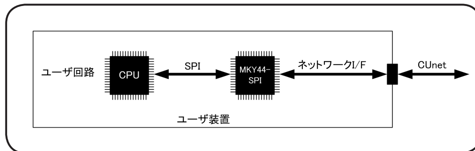
図 1.1 MKY44-SPI を搭載した CUnet ステーション図 (MEM ステーション)
