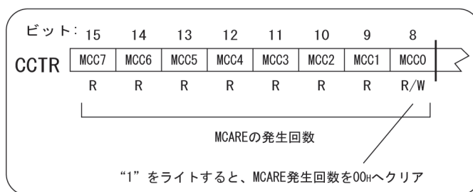
図 5.30 CCTR の MCARE 発生回数
