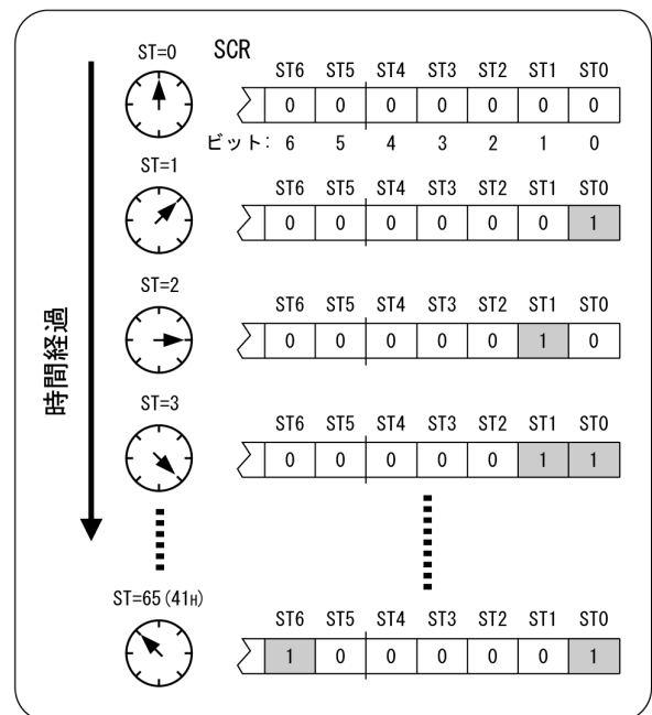
図 5.4 SCR のビット 0 ~ 6 が示すステーションタイム
