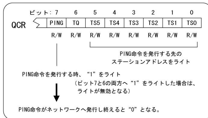
図 5.32 PING 命令の発行
