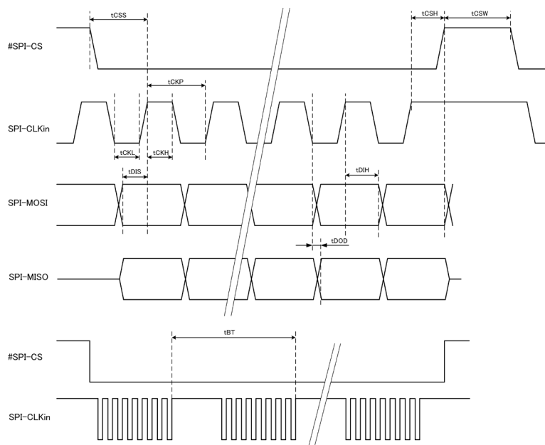
図 4.4 SPI タイミング図
