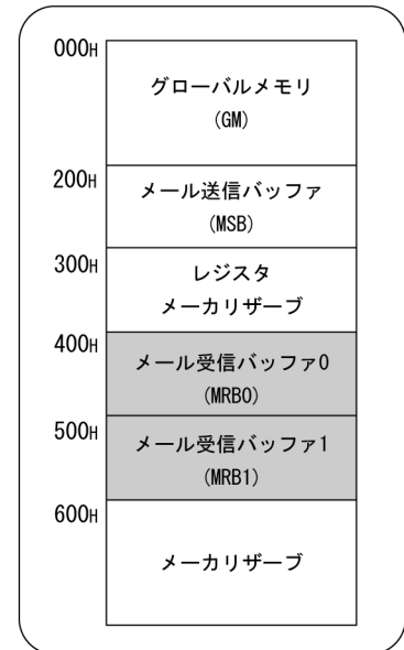
図 5.16 メール受信バッファ
