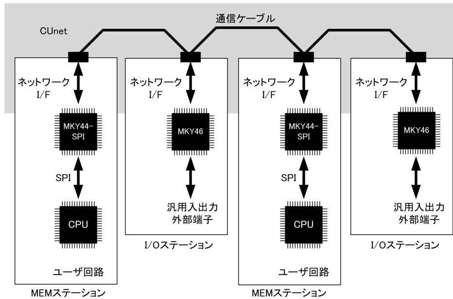
図 1.4 I/Oステーションを接続したCUnet構成
