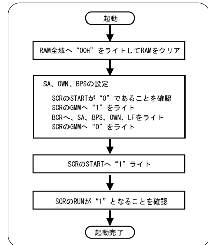
図 5.1 起動のアルゴリズム
