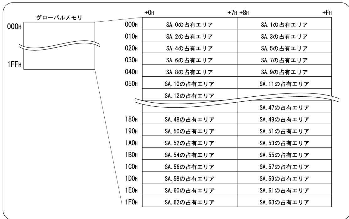
図 5.5 グローバルメモリ
