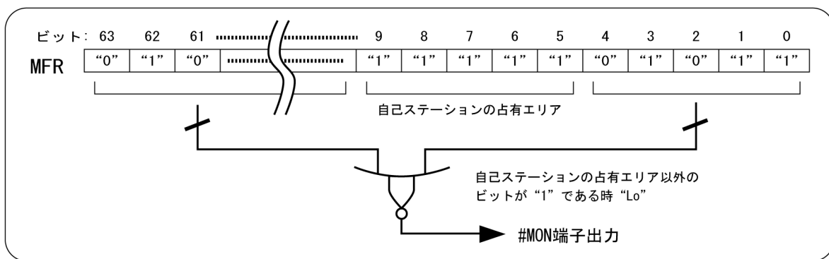
図 5.31 #MON 端子への出力例
