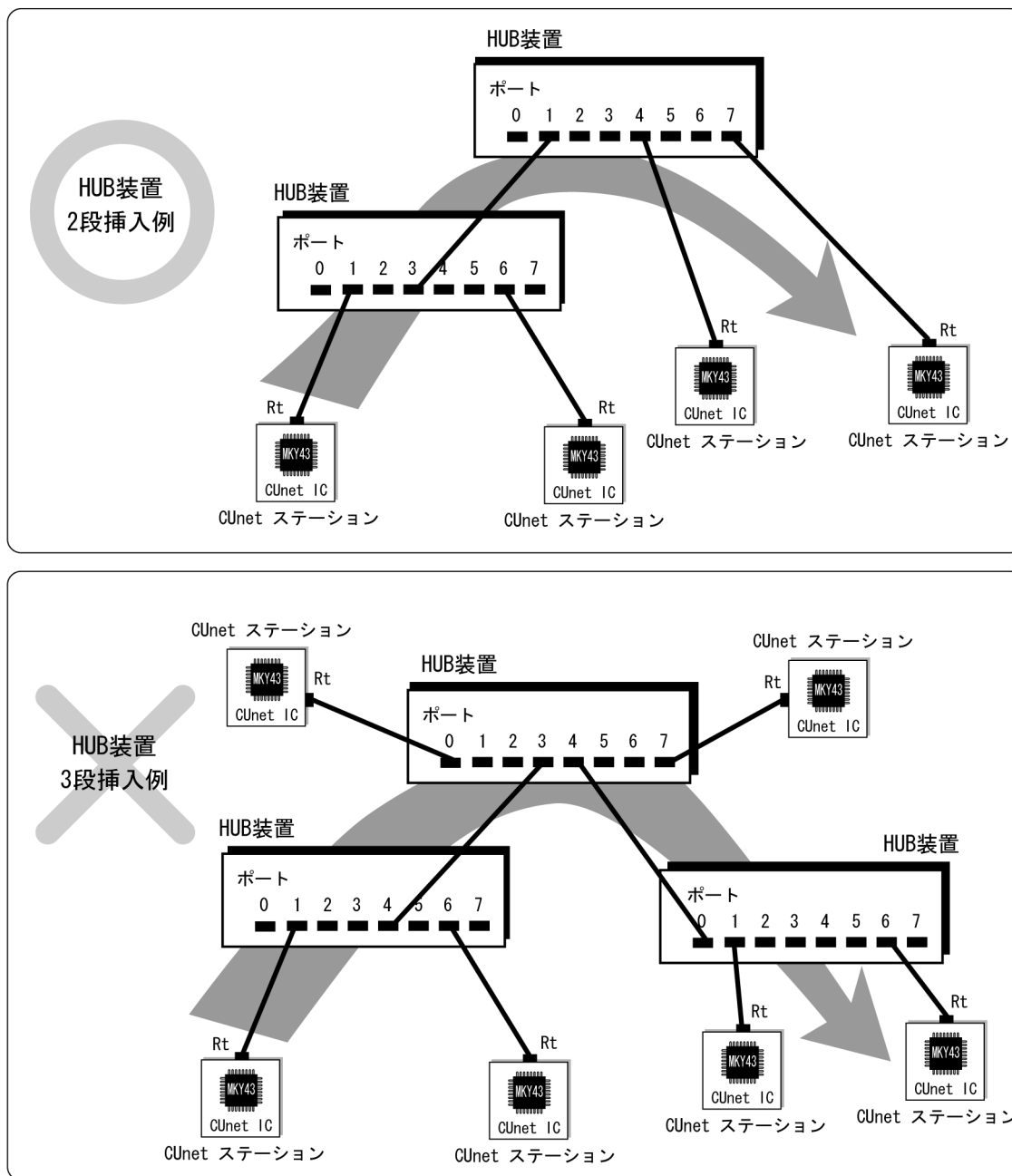
図 5.34 HUB 挿入可能段数
