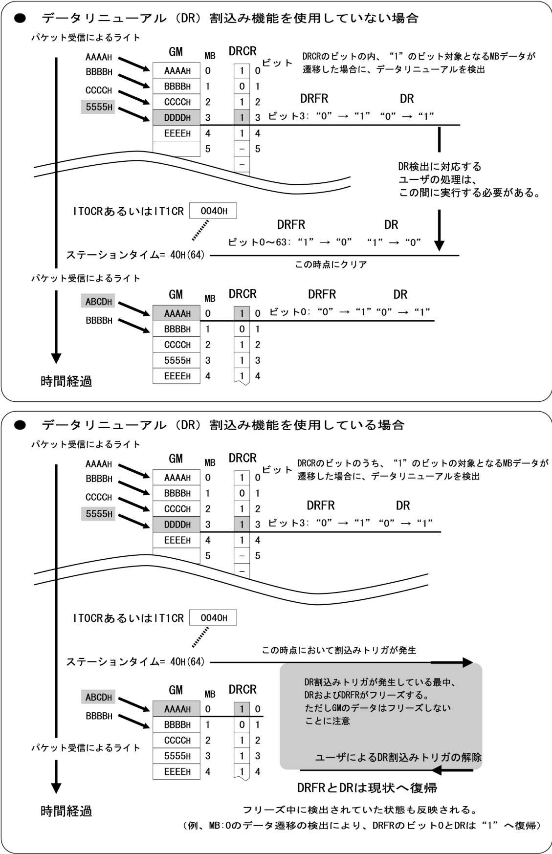
図 5.15 時間経過に対するデータリニューアル検出の概要
