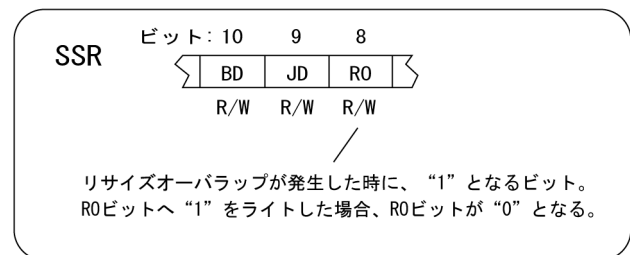
図 5.26 SSR の RO ビット
