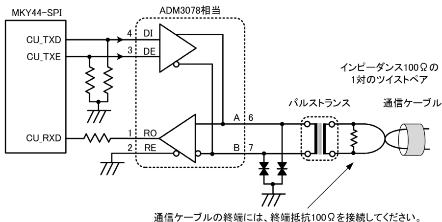
図3.1 推奨ネットワーク接続図
