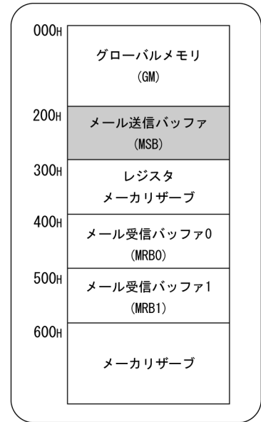
図 5.20 メール送信バッファ
