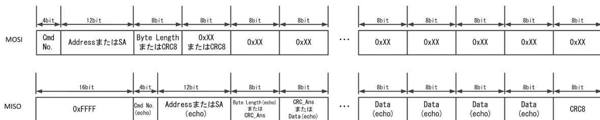
図 4.2 SPI コマンド (Read) 基本フォーム
