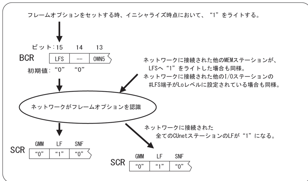
図5.35 フレームオプションの設定
