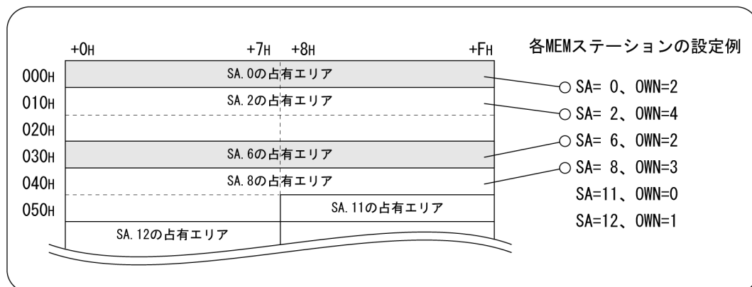
図 5.6 占有エリアの拡張
