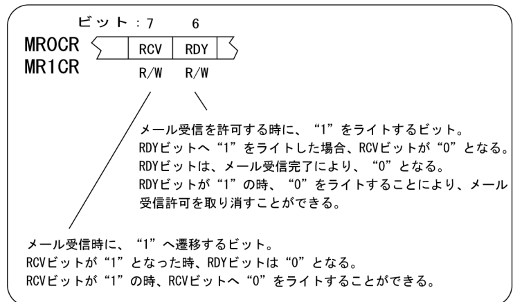
図 5.17 メール受信許可
