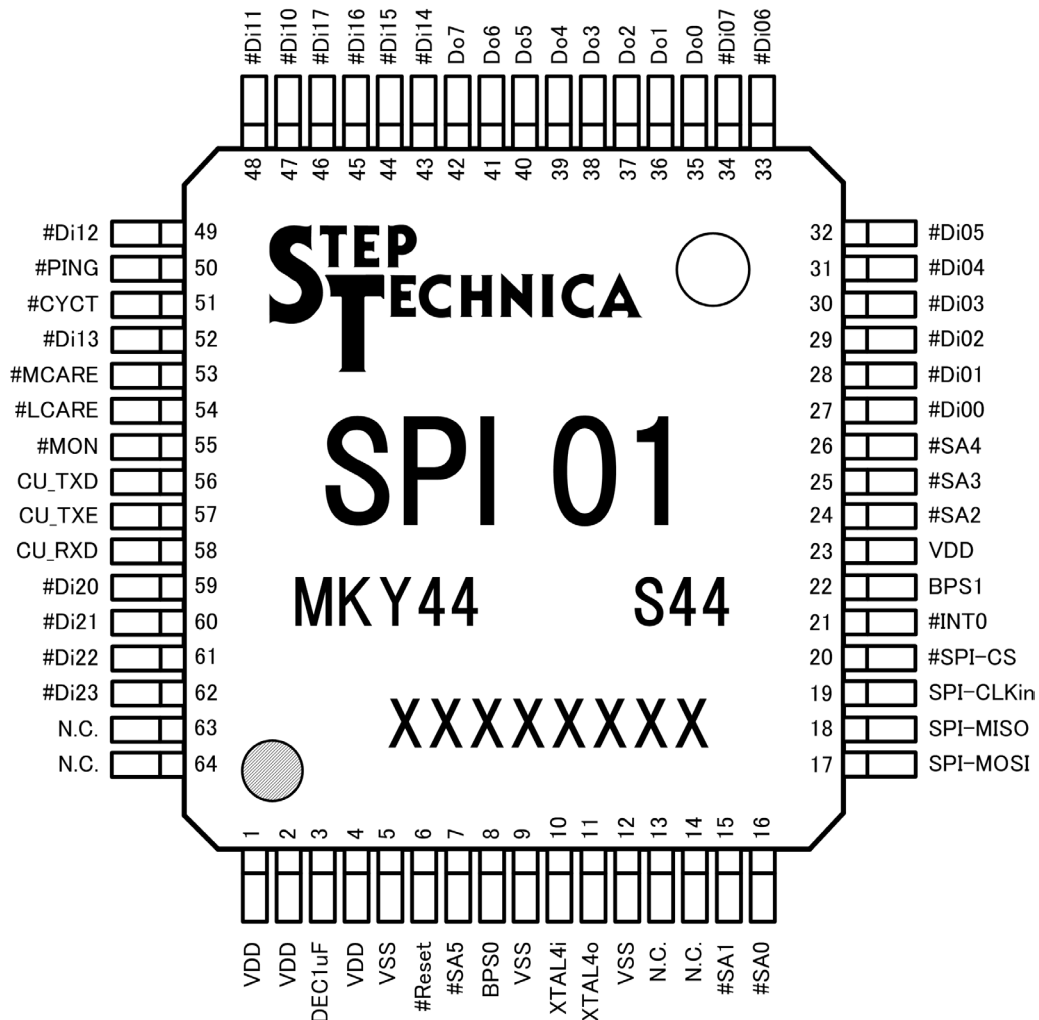
図2.1 端子配列図 (Top View)
