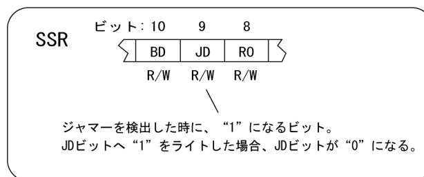
図 5.28 SSR の JD ビット
