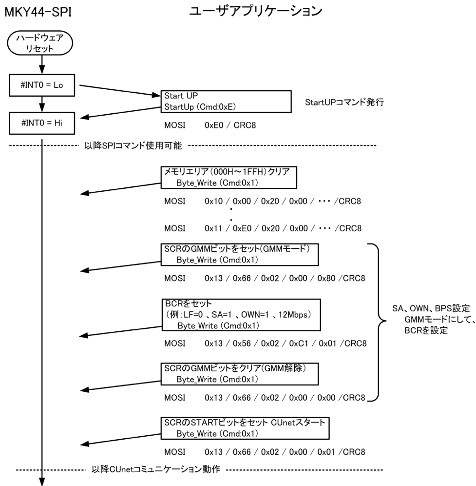
図 4.3 起動時及びリセット時の手順
