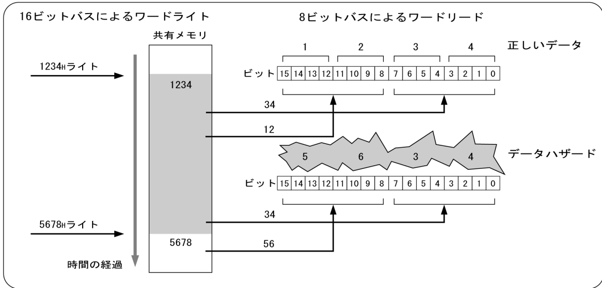
図 5.7 データハザード発生メカニズム
