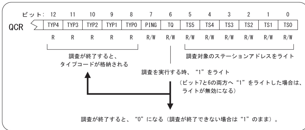
図 5.33 各MEMステーションのモード調査
