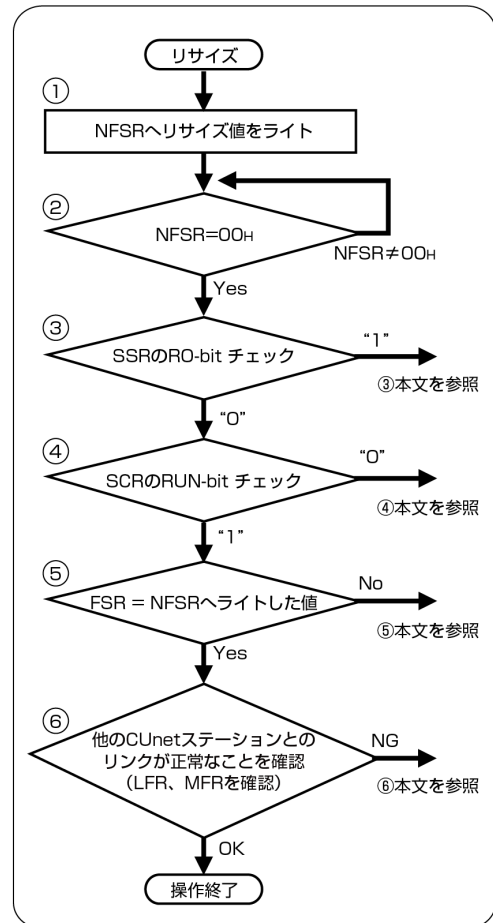
図 5.25 リサイズの実行
