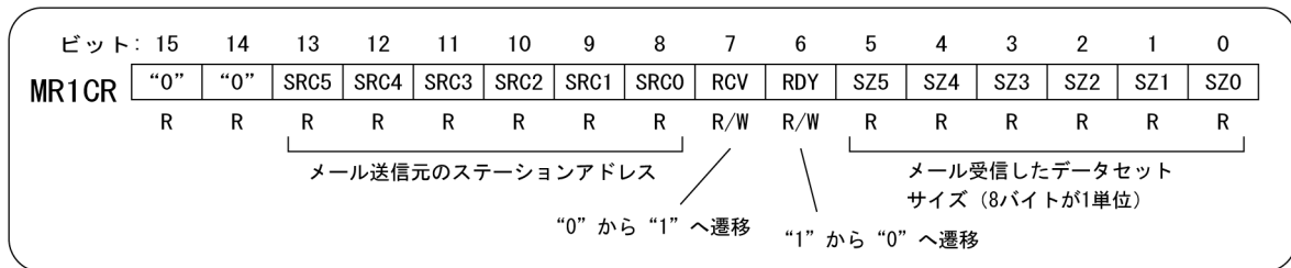
図 5.19 MRB1 へデータセットを格納した時の MR1CR
