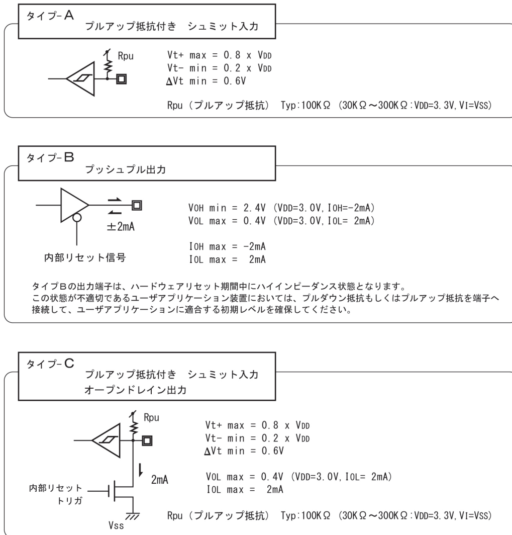
図 2.2 タイプ別端子定格図
