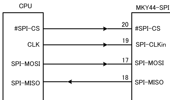
図 3.2 SPI 接続図
