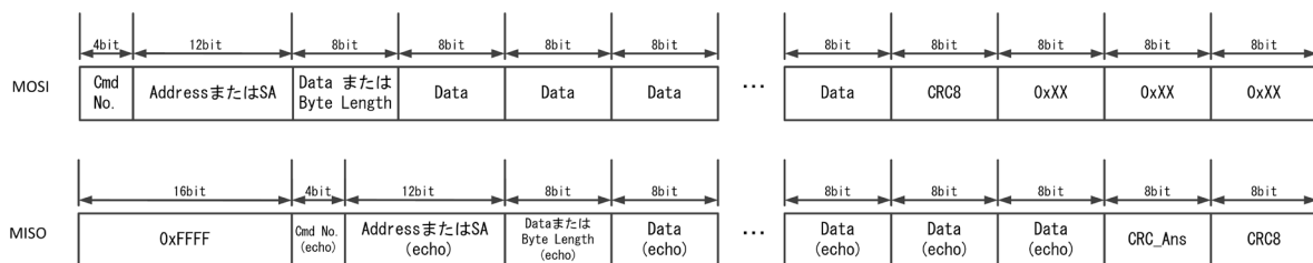
図 4.1 SPI コマンド (Write) 基本フォーム
