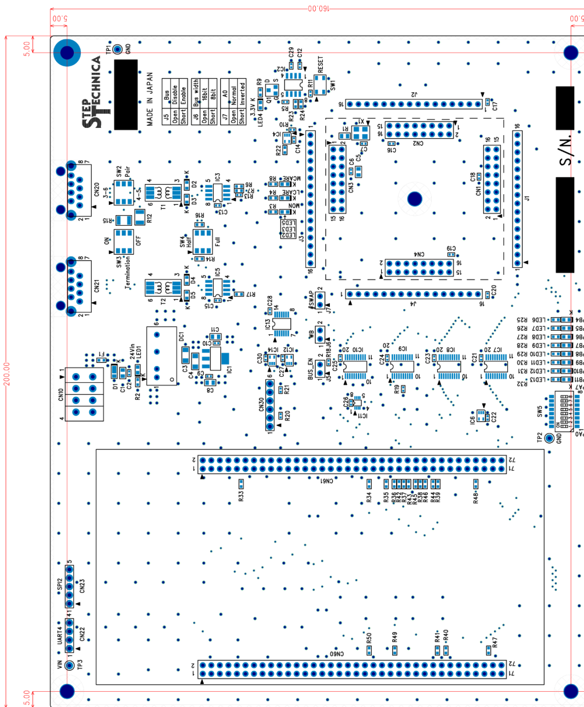
图 5-2 IB-43 基板外形寸法图
