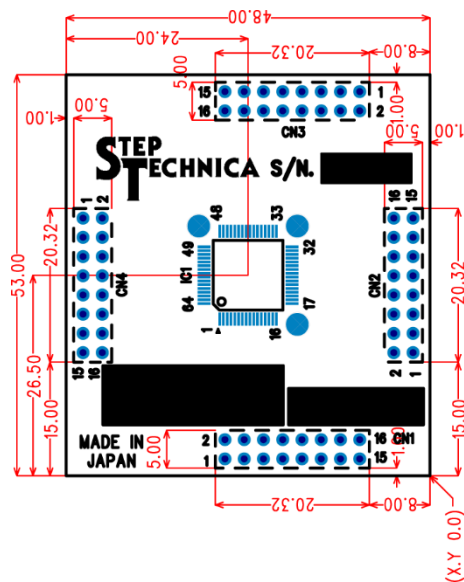
図 5-1 DB-36 基板外形寸法図
