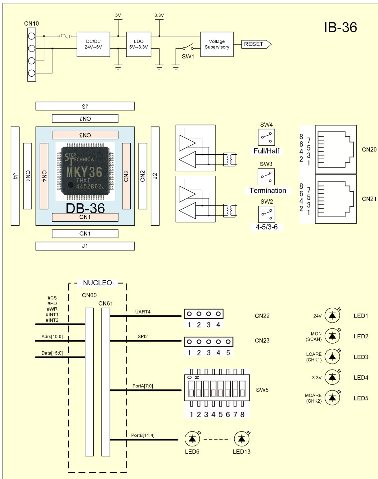
図 3-1 ブロック図
