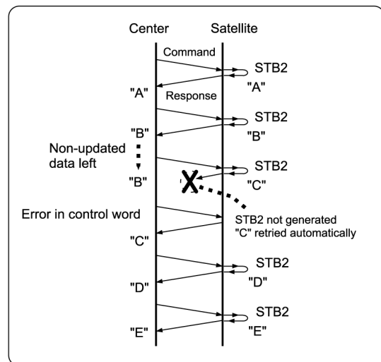
Fig. 4.5C Handshaking Enabled
