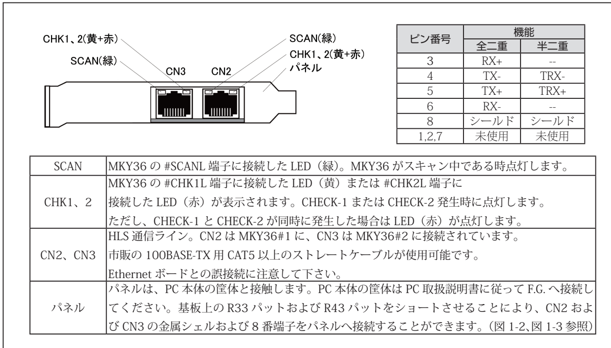
図 1-1 パネル概観
