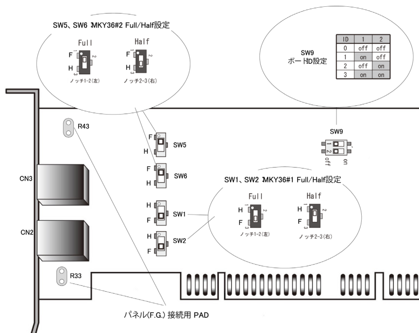
図 1-3 HLSB-36PCI2 ボードの設定
