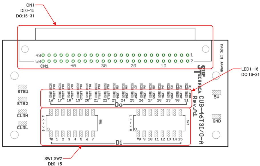
CUB-46T3I/O-A 基板 外観図
