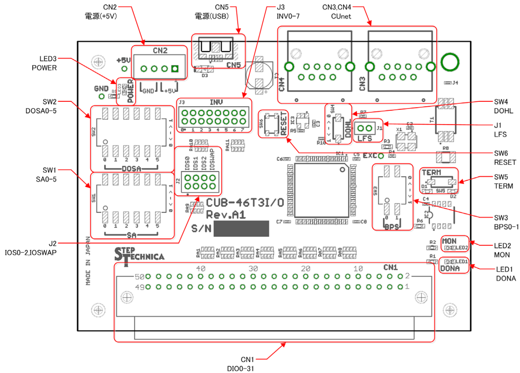
CUB-46T3I/O 基板 外観図
