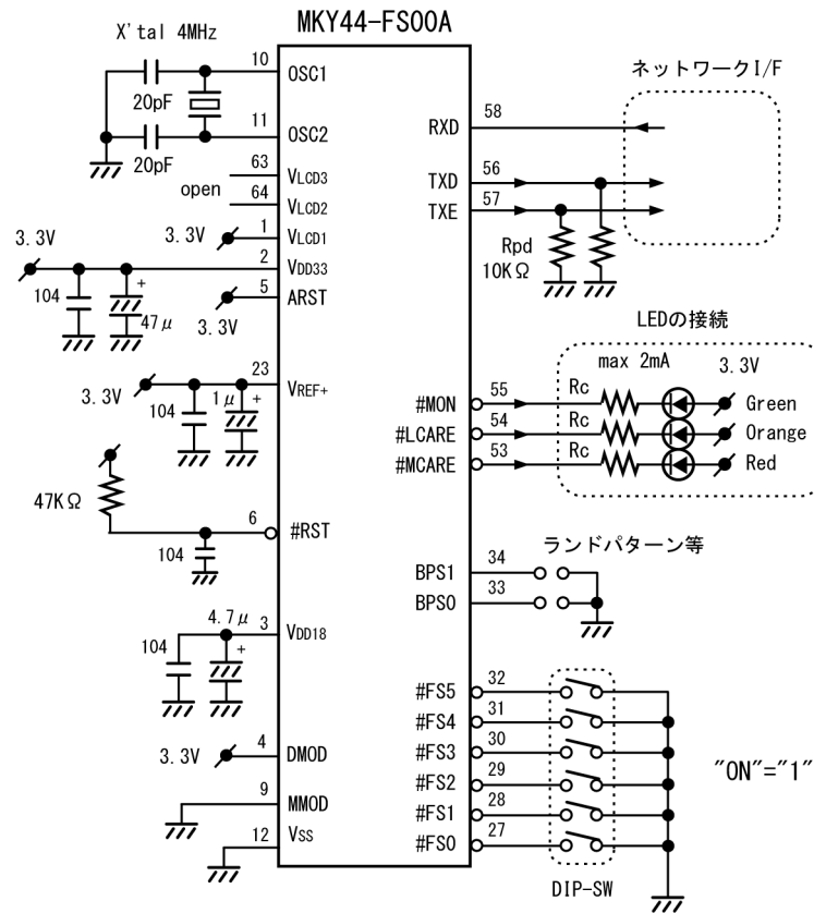
MKY44-FS00A 標準推奨の接続
