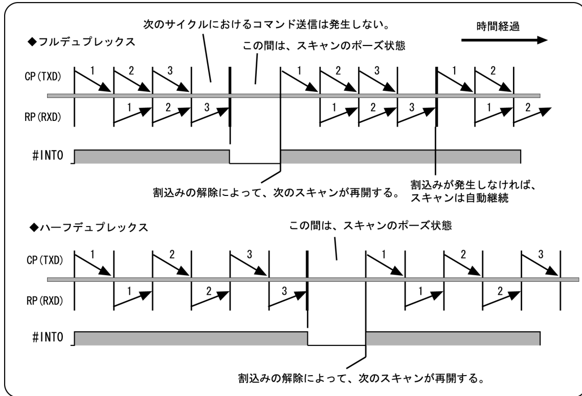
図2. 19 DR2の動作
