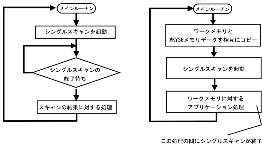
図2.5 シングルスキャン利用のアルゴリズム例
