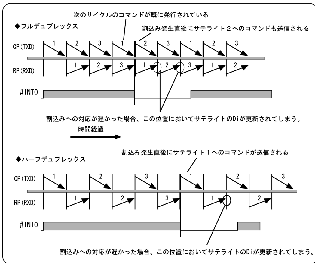
図2.18 DR1のデータ遷移継続状況
