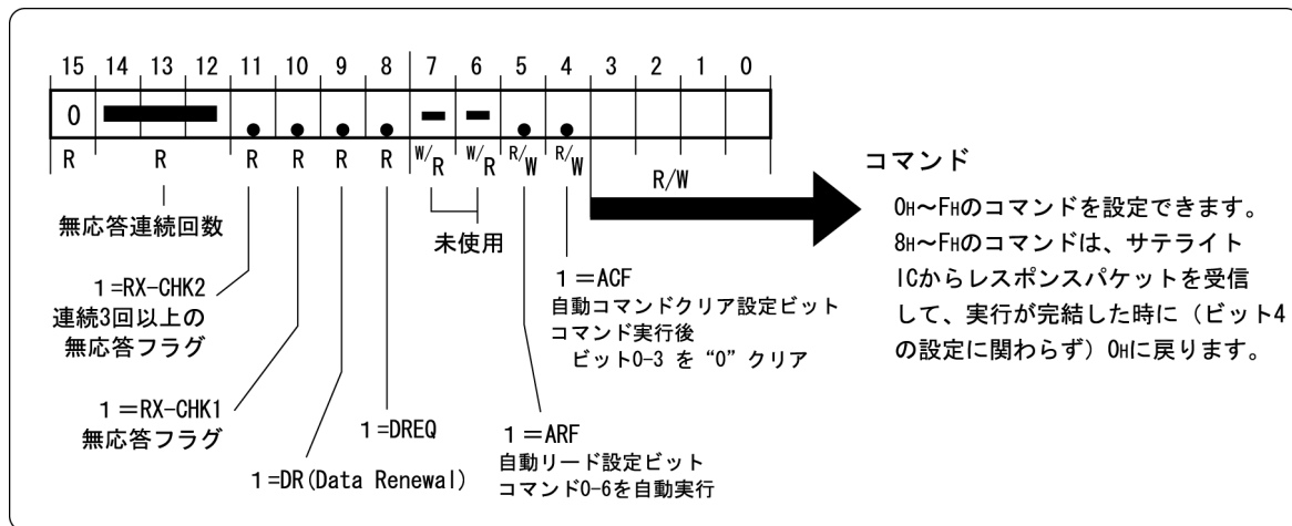
図2.7 コントロールワードの構成
