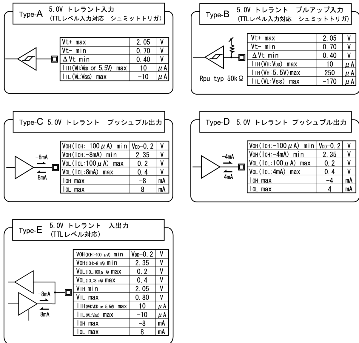
図3.2 MKY36の入出力回路形式における端子電気的特性
