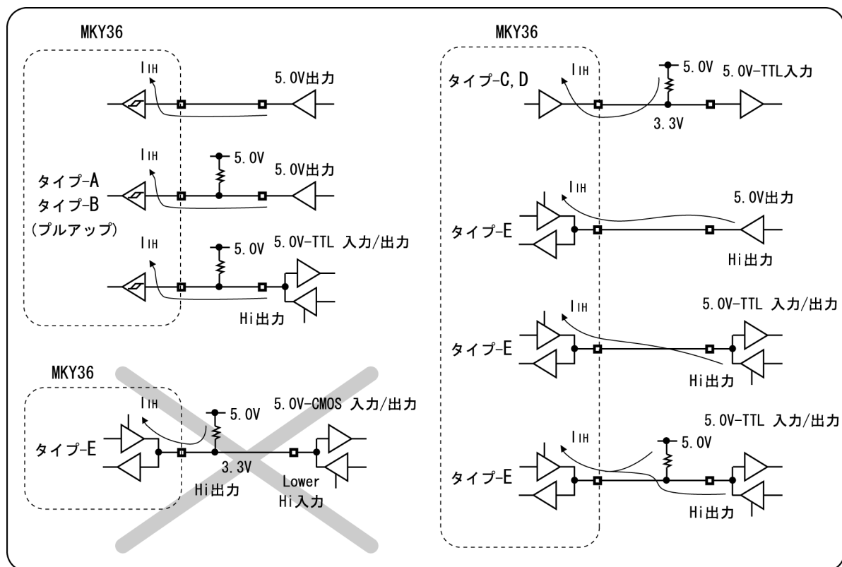
図4.1 リークの生じる接続
