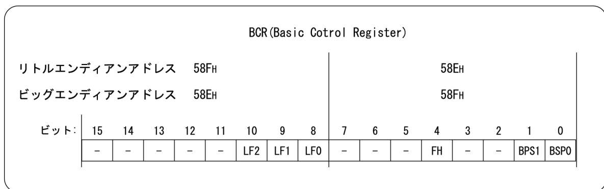
図4.4 エンディアンによるバイトアクセスのアドレス相違
