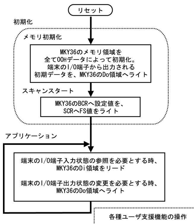
図1.1 MKY36の操作
