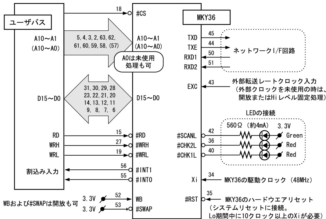
図4.6 16ビットユーザバスとの接続
