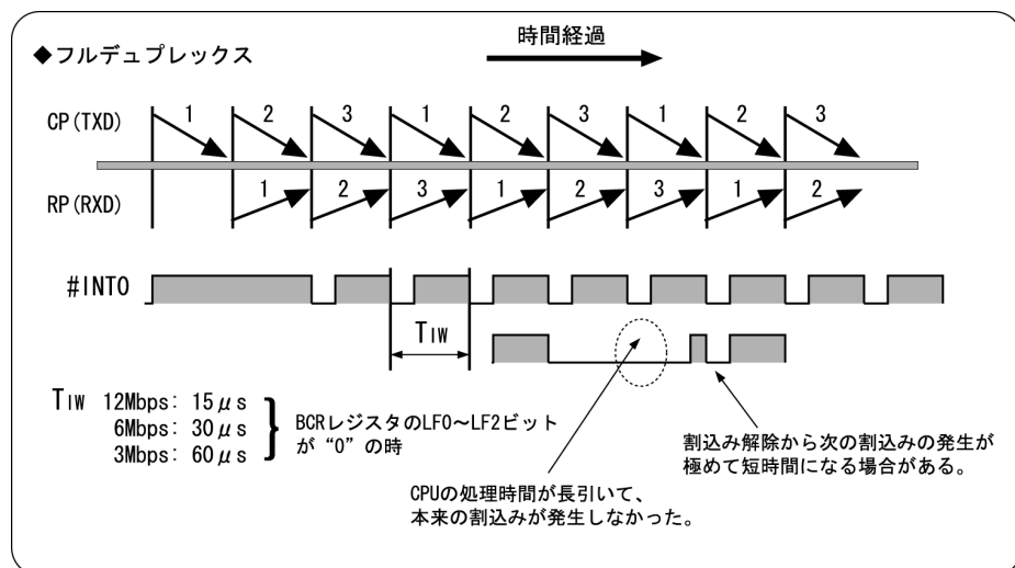
図2.16 DR0の割り込みを発生しない
