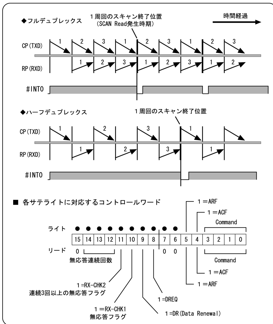
図2.17 DR1の動作
