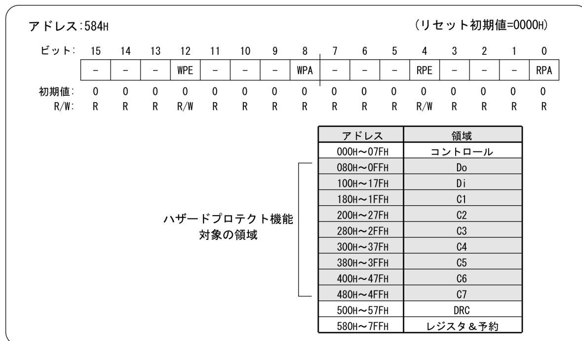
図2.9 HPRおよびHP機能の対象アドレス
