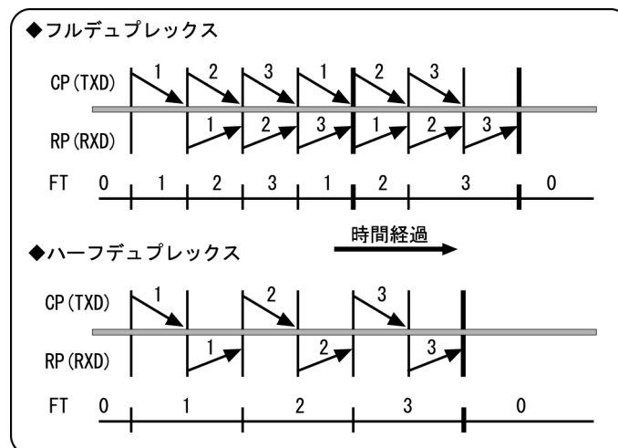
図2.4 FT値の推移
