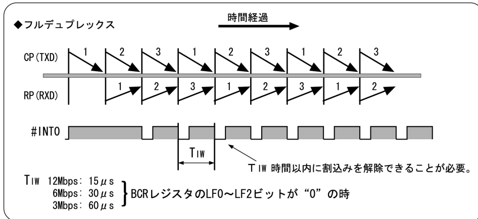
図2.15 DR0の動作
