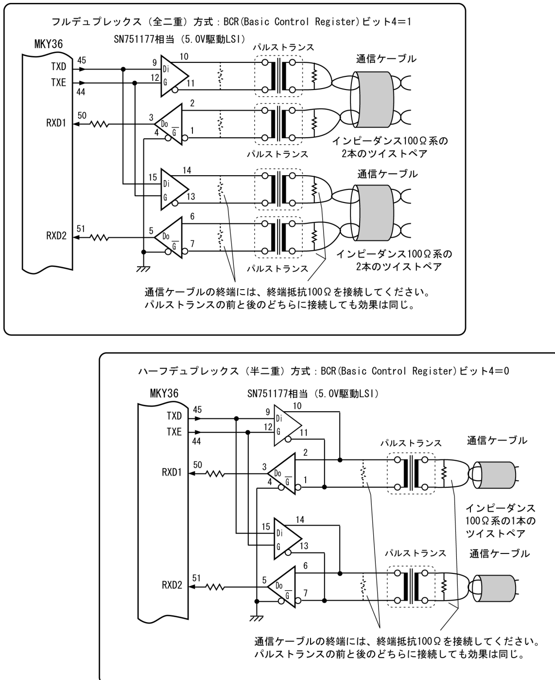
図4.3 推奨のネットワーク接続
