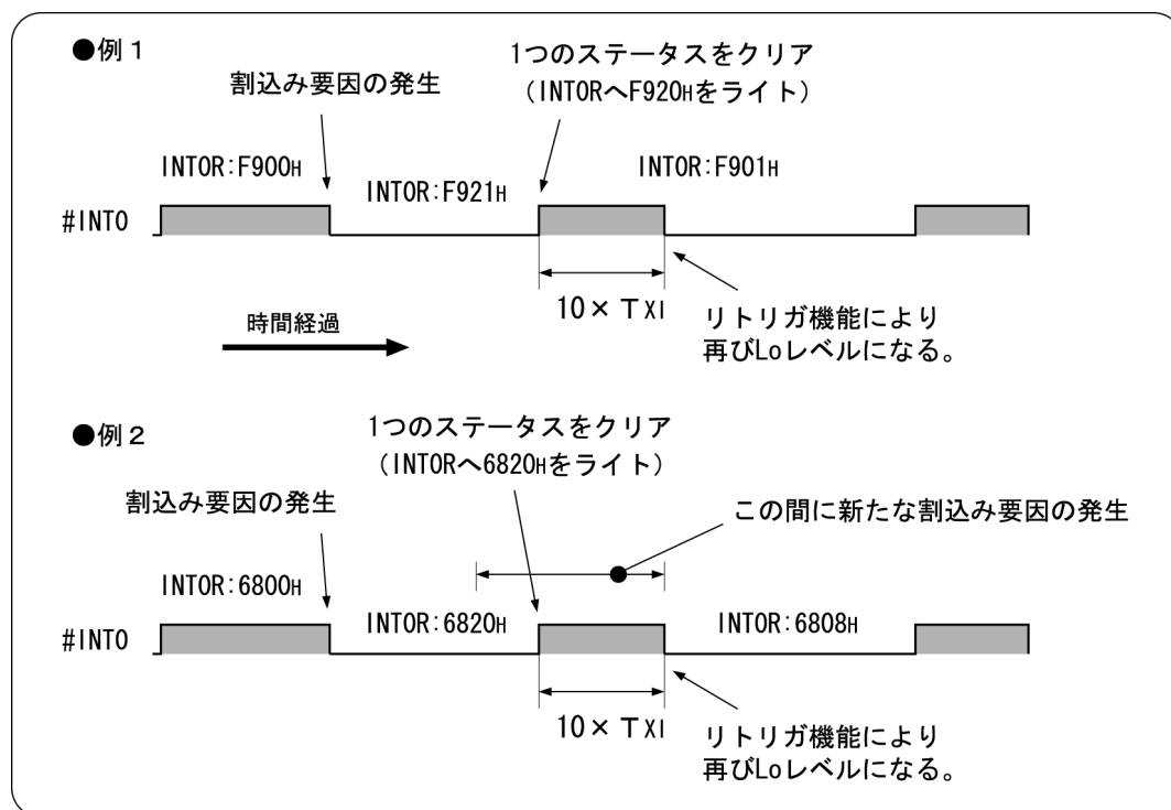
図2.13 リトリガ機能
