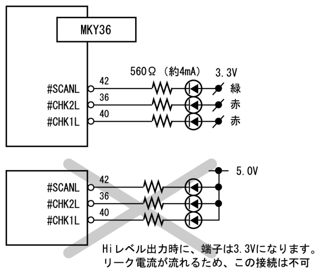
図4.7 LEDの接続
