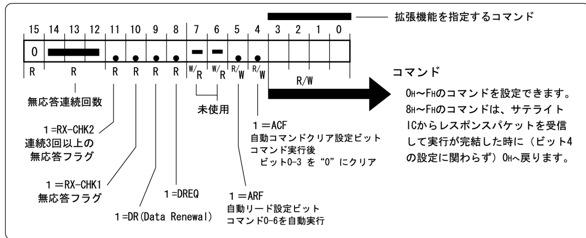
図2.8 拡張機能を指定するコマンド
