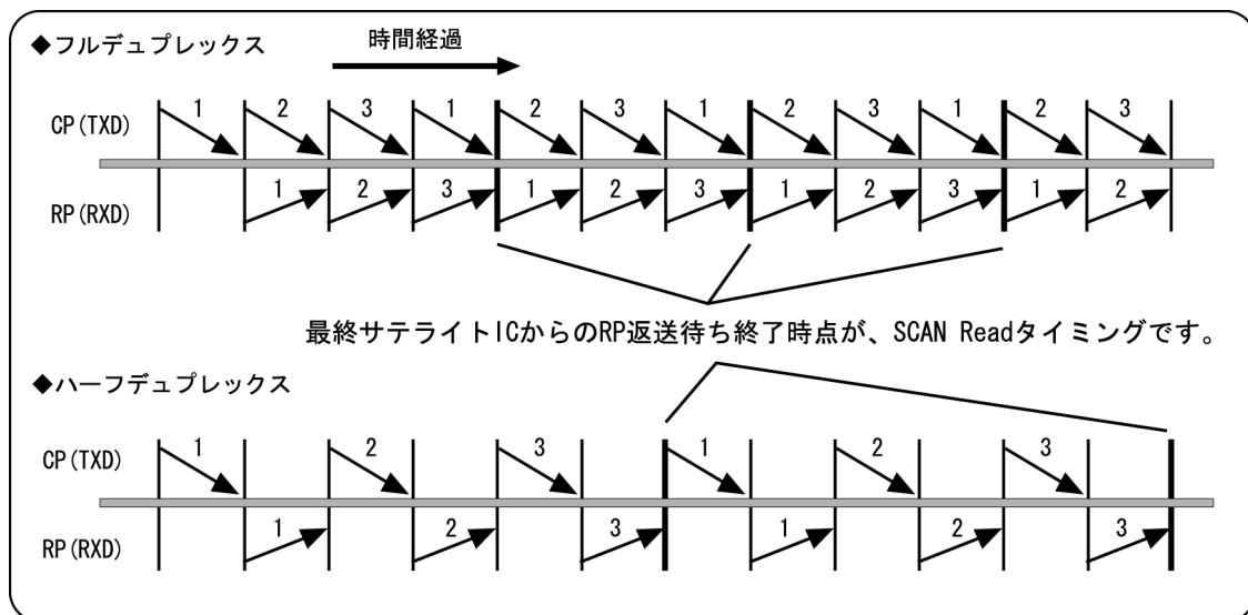
図2.6 スキャンリードのタイミング位置
