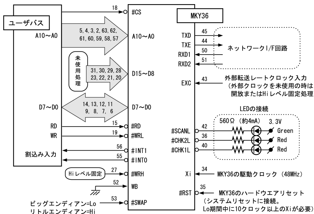
図4.5 8ビットユーザバスとの接続
